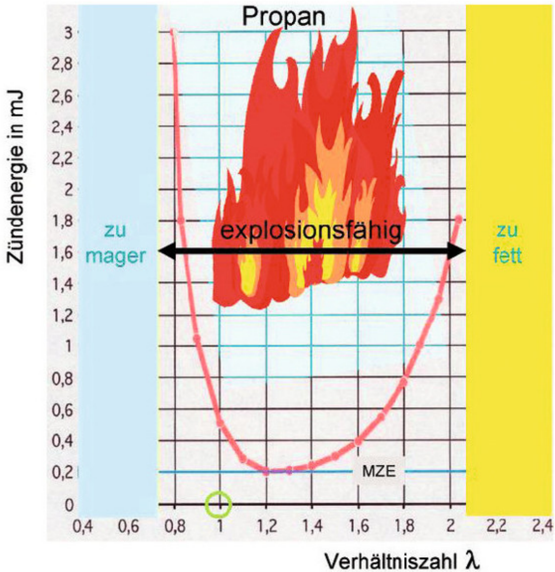
Abbildung 1: Abhängig von der Dichte des Brenngases benötigten Gemische außerhalb der stöchiometrischen Verhältniszahl \lambda=1 eine höhere Energie zur Zündung. (Bild: Elstatik)
